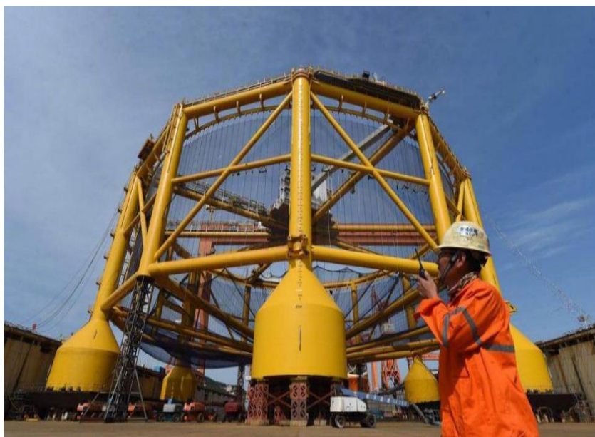
武船集团为挪威萨尔马集团制造的世界首座深海渔场“海洋渔场一号”
