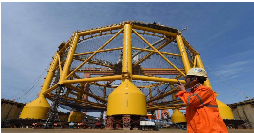
中船重工武船集团为挪威萨尔马集团制造的世界首座深海渔场“海洋渔场一号”
